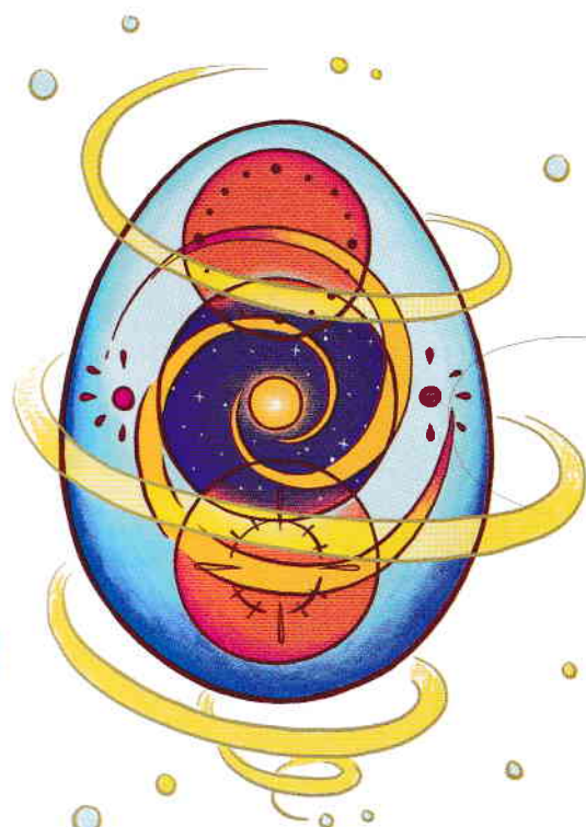
ou cosmic
